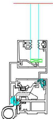
Détail B
